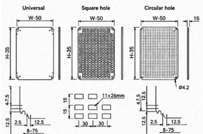
5.2) PLACAS DE MONTAJE / PATRONES DE PERFORACIÓN (mm)
