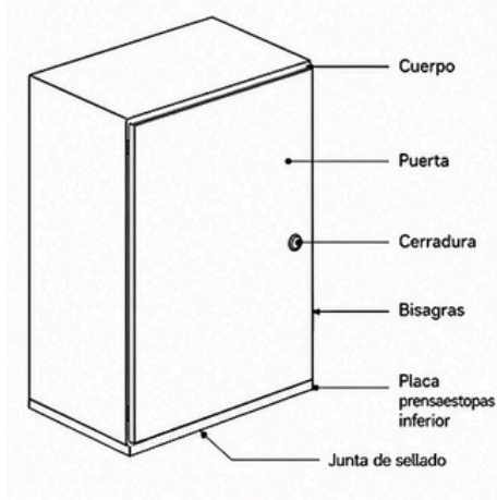
1) VISTA ISOMÉTRICA GENERAL
